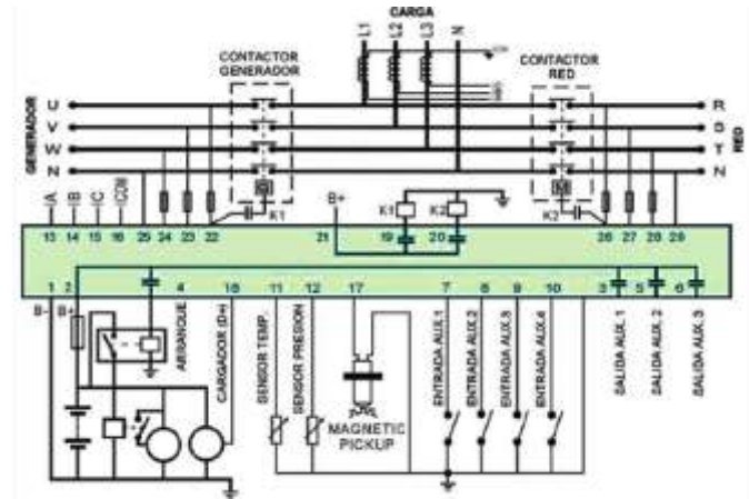
Plano de conexionado controlador HGM42010
